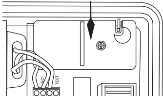
Instalovaný a připojený SLHUBRF modul
