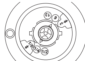
Pro nastavení čidla srážek stlačit a pootočit
