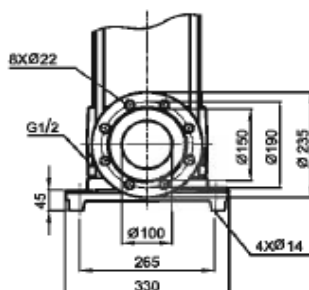
Příruba (DIN) PN16 / DN100
