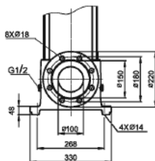
Příruba (DIN) PN16 / DN100
