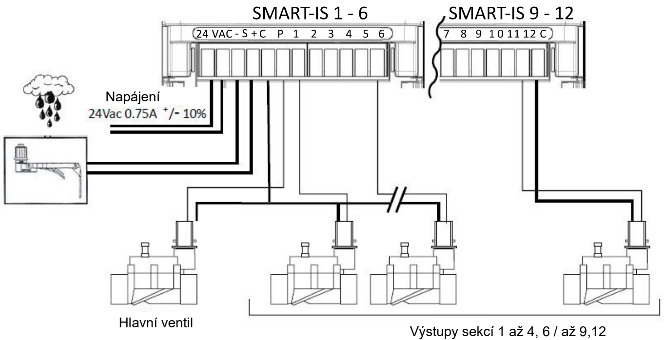
Zapojení s čidlem srážek
